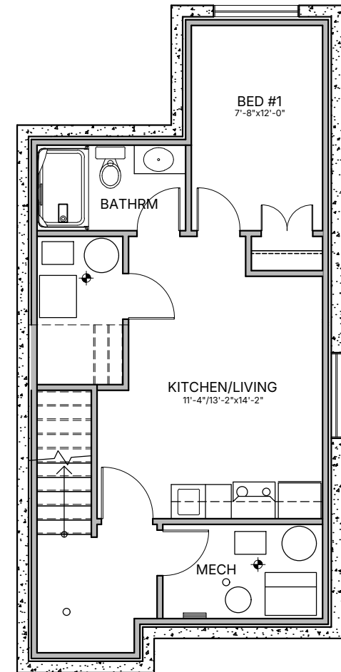
OPTIONAL BASEMENT SUITE LAYOUT - 656 sq.ft.
